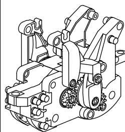
齒輪箱 Gear Box
