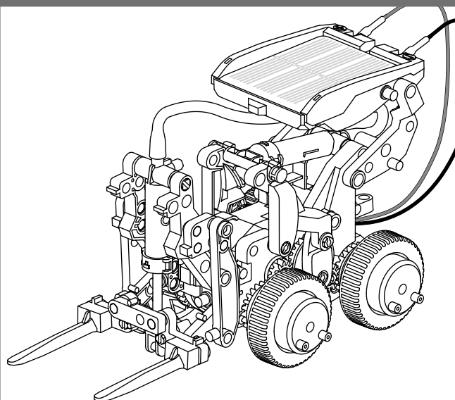
齒輪箱 Gear Box
