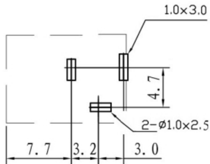
线路板安装尺寸示意图
