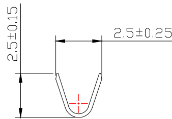
A - A
