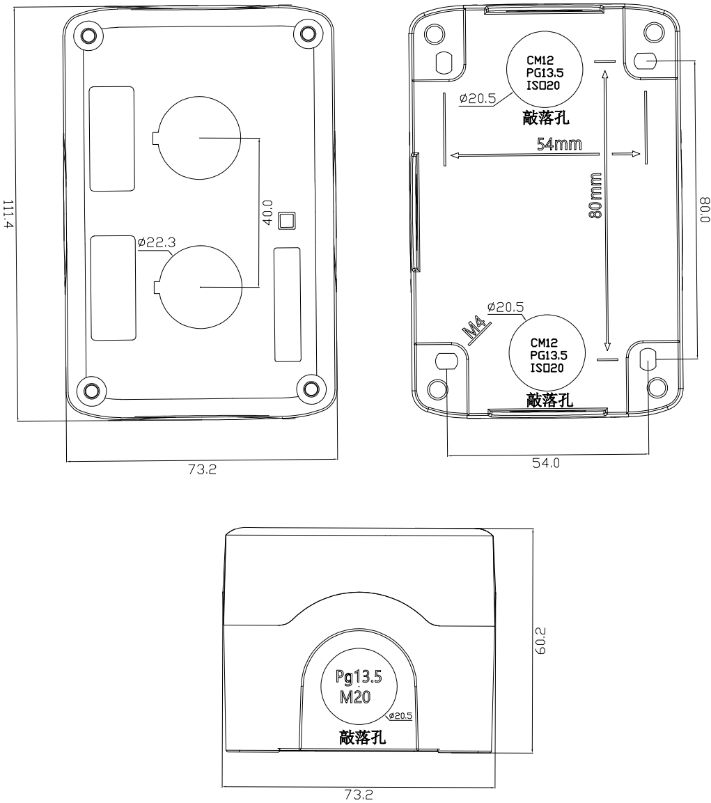
尺寸图（公差：±0.2）
