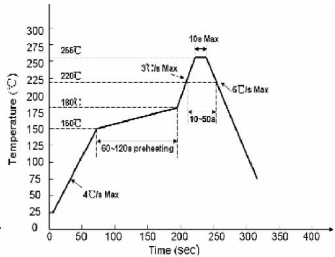
無鉛製程
