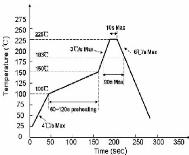
有鉛製程
